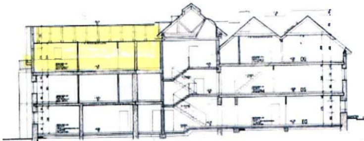
Schnitt
