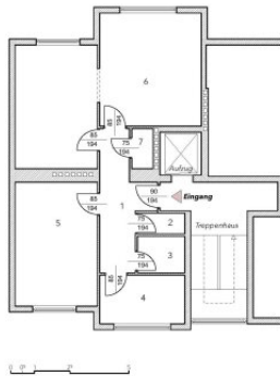
Wohnungsgrundriss Bestand
